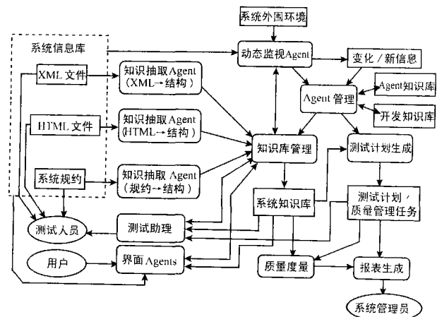
图 3 MAISGE - AquIS 结构示意图
