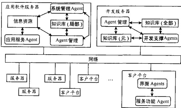
图 2 多 Agent 软件生长环境 MAISGE
